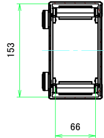
A-A (1:4.5)
